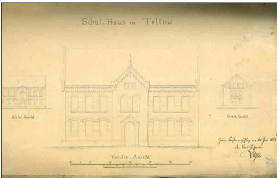
Die Bauzeichnung des Bau-Inspectors Vogel, Kreisarchiv Potsdam-Mittelmark
